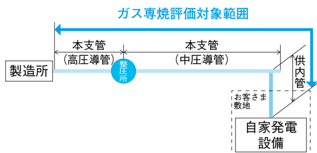
図1 本支管／供内管及び評価対象範囲の概念図
